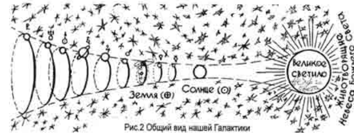
Рис.2 Общий вид нашей Галактики
